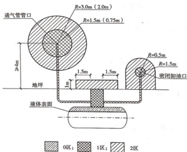
图 3 埋地卧式汽油储罐爆炸危险区域
